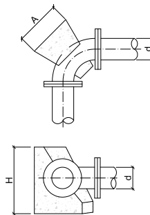
DETALL COLZE 90° TIPUS S/E
