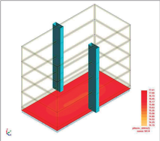
COMBINACIONS D'HIPÒTESIS ELS- REACCIONS DEL SÒL
