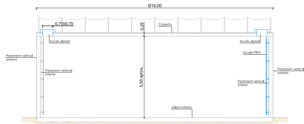
Secció A-A'
