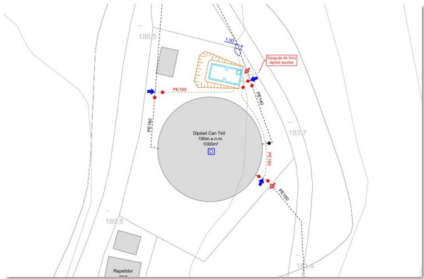
Esquema instal·lacions previstes a Can Tiril
