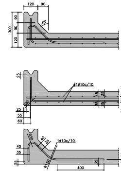
DETALL JUNTA ENTRE ANELLS E:1/5
